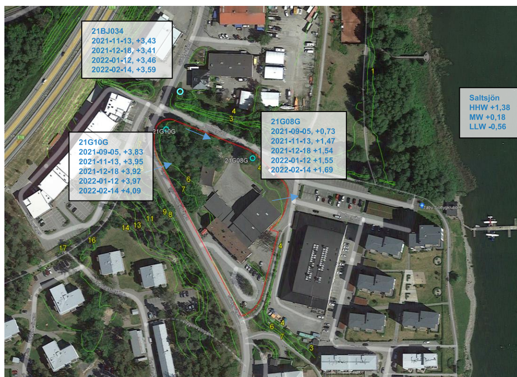
Figur 8. Uppmätta grundvattentrycknivåer samt bedömning av grundvattnets strömningsriktning. Angivna grundvattentrycknivåer är uppmätta från augusti 2021 – februari 2022. Grundvattennivån ska förutsättas variera med årstid och nederbörd.
