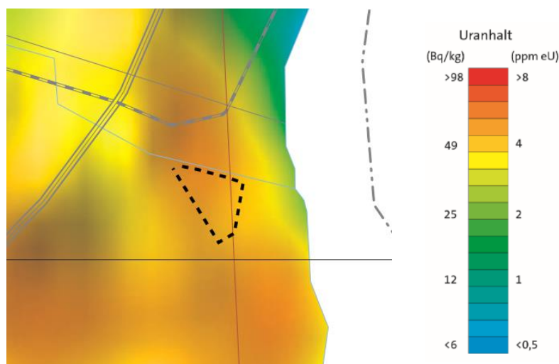
Figur 9. Uranhalten i mark enligt SGU:s gammaspektrometriska mätningar.
